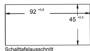
Schalttafel Ausschnitt
