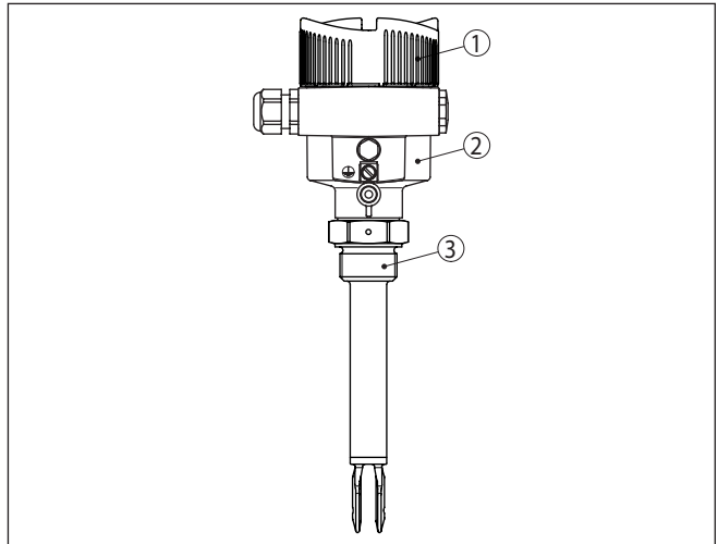
Fig. 1: SITRANS LVL200E
