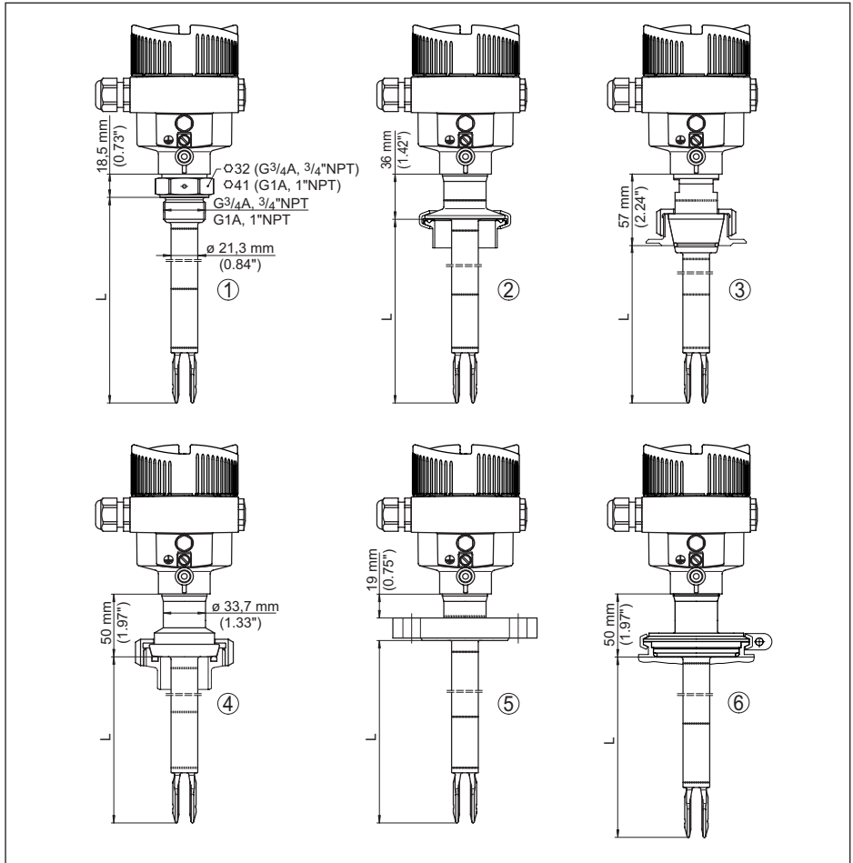
Fig. 36: SITRANS LVL200E
